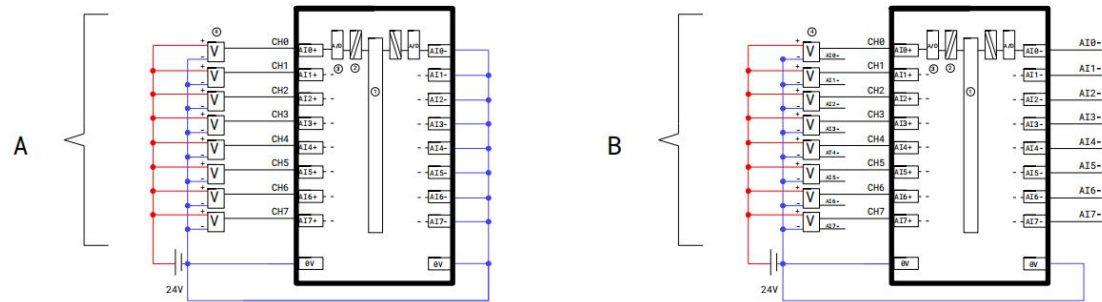
MXIO 431-1KF00-0AA0 8通道模拟量电压输入
