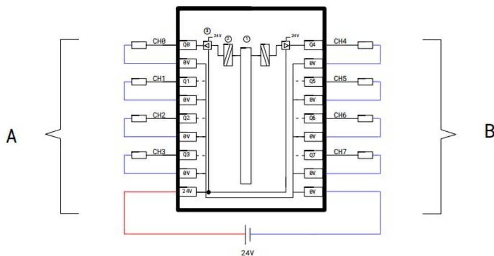
MXIO 422-1BF01-0AA0 数字量8路源型输出 源型输出
