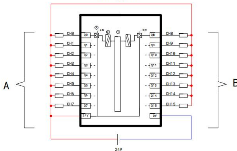
MXIO 422-1BH00-0AA0 数字量16路漏型输出 漏型输出
