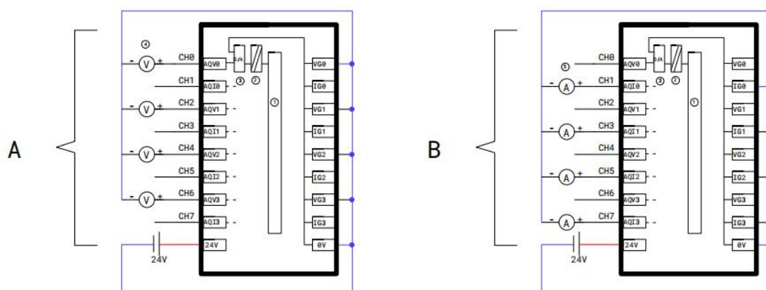
MXIO 432-1KD02-0AA0 4路模拟量输出(电压电流)
