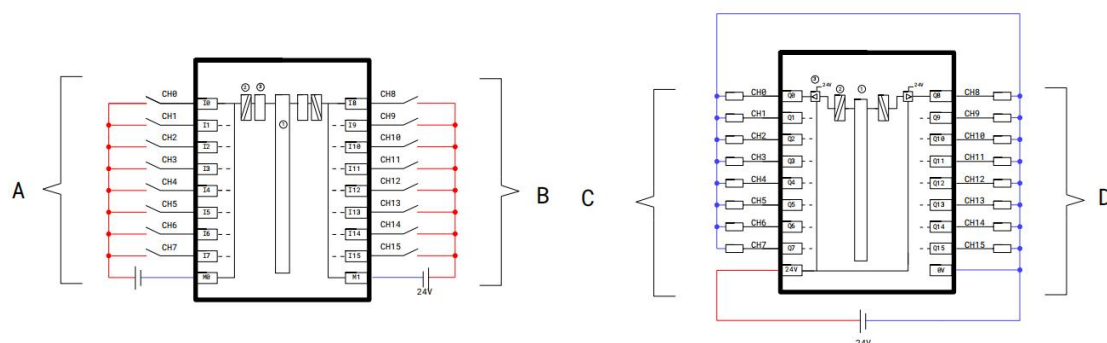
MXIO 423-1BL01-0AA0 数字量16路输入 数字量16路输出(源型) 源型输入 源型输出
