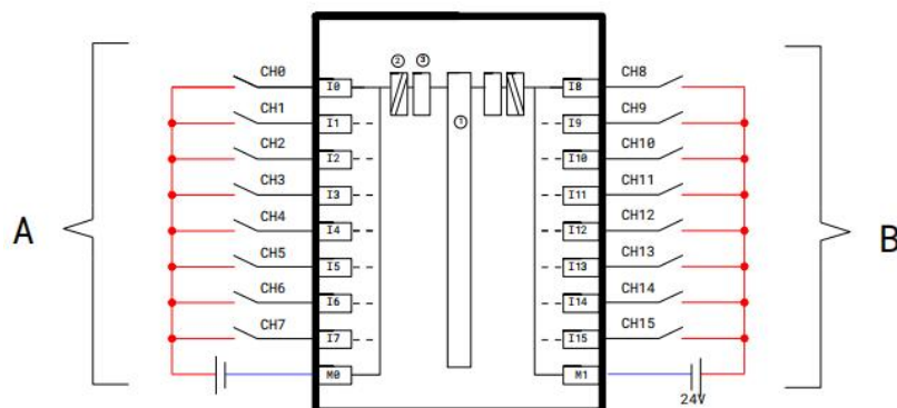
MXIO 421-1BH00-0AA0 数字量16路源型输入 源型输入
